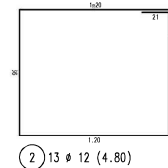
Bewehrung im Schnitt 1-1 - M 1:20
