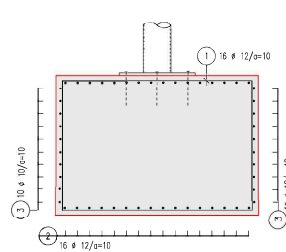
Bewehrung im Schnitt 1-1 - M 1:20
